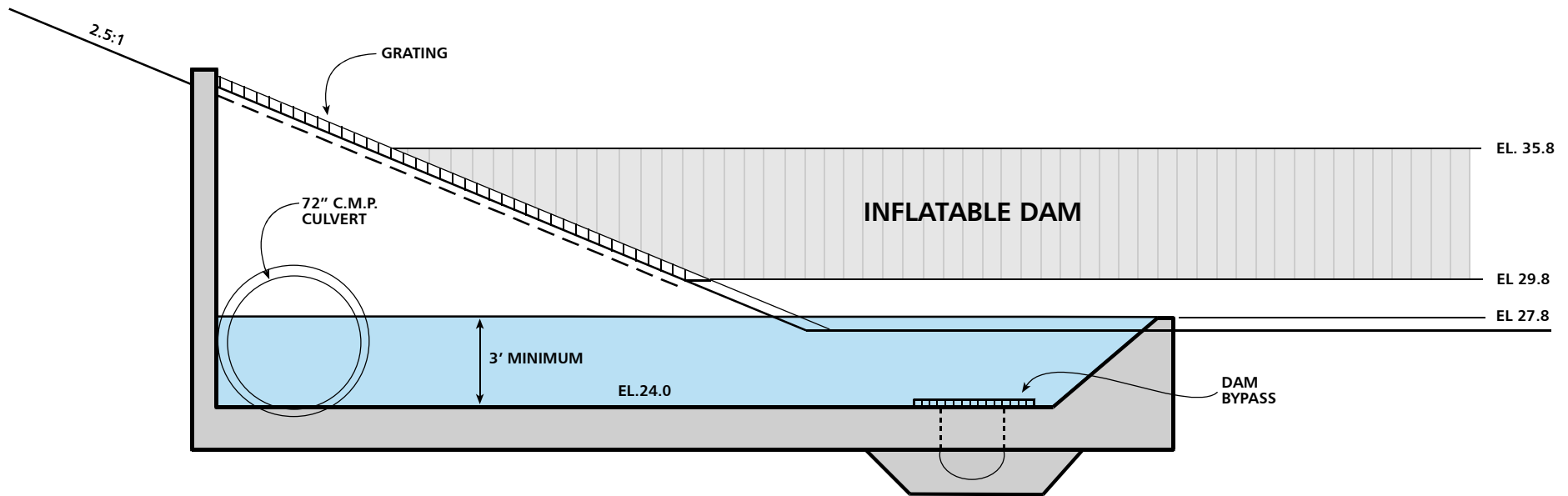
SECTION A-A
